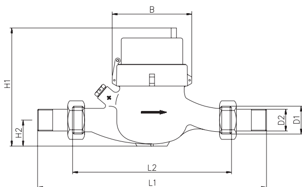
Dimensions IMF
