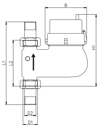
Abmessungen IMF-ST
