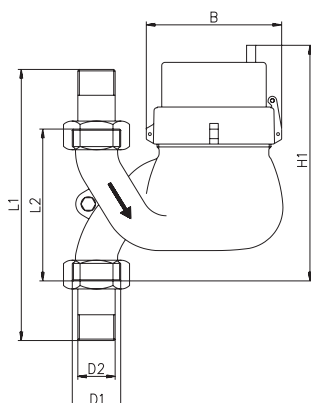
Abmessungen IMF-FA
