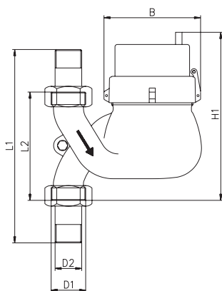
Dimensión IMF-FA
