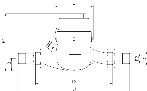
Dimensioni IMF
