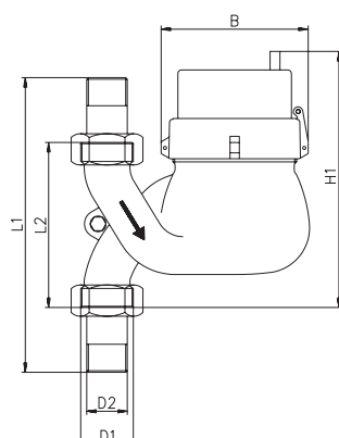
Dimensions IMF-FA
