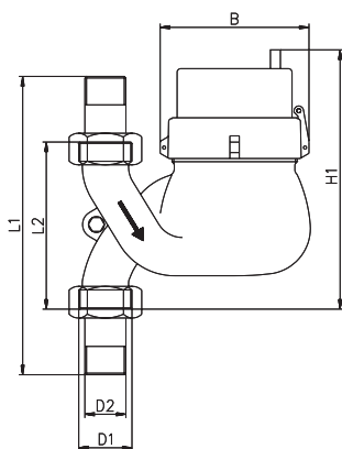
Dimensions IMF-FA
