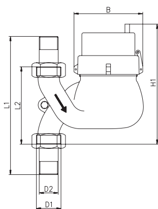
Dimensioni IMF-FA (a flusso discendente)
