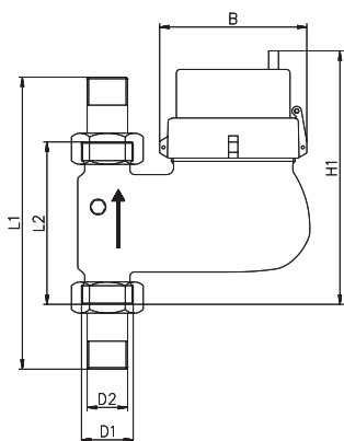
Dimensions IMF-ST
