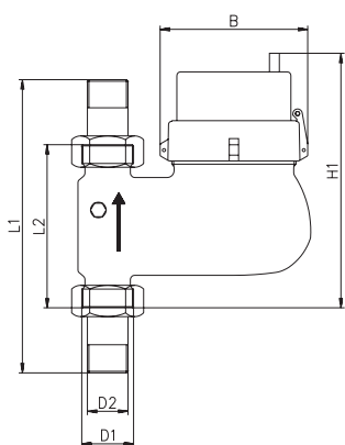
Dimensioni IMF-ST (a flusso ascendente)
