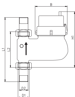
Dimensions IMF-ST
