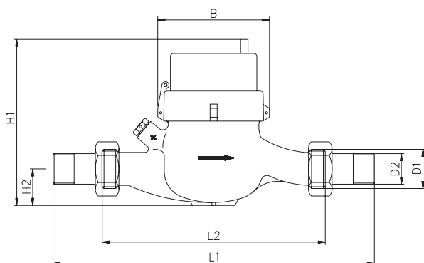
Abmessungen IMF
