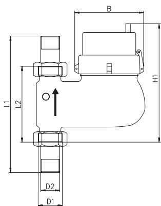
Dimensión IMF-ST
