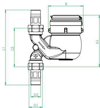
Dimensions
